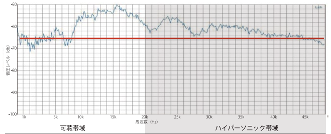
Egretta 自社開発ハイルドライバー方式トゥイーターの周波数特性
